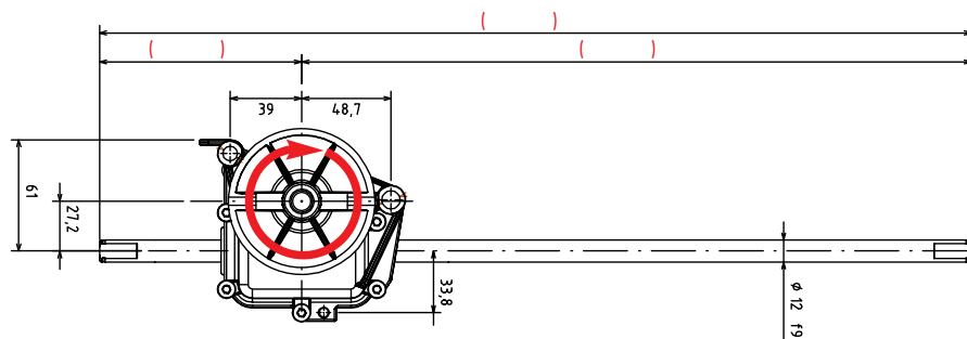
Sistema Trazione Brevettato - Patented Traction System
